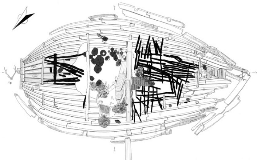
〈그림 11〉 마도 3호선 선내 유물 배치도 (국립해양문화재연구소 2012c, 80).
